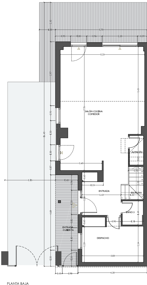
PLANTA BAJA
