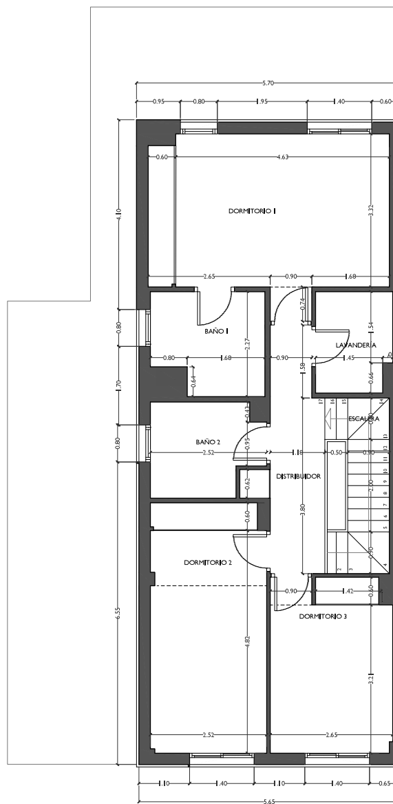
PLANTA PRIMERA
